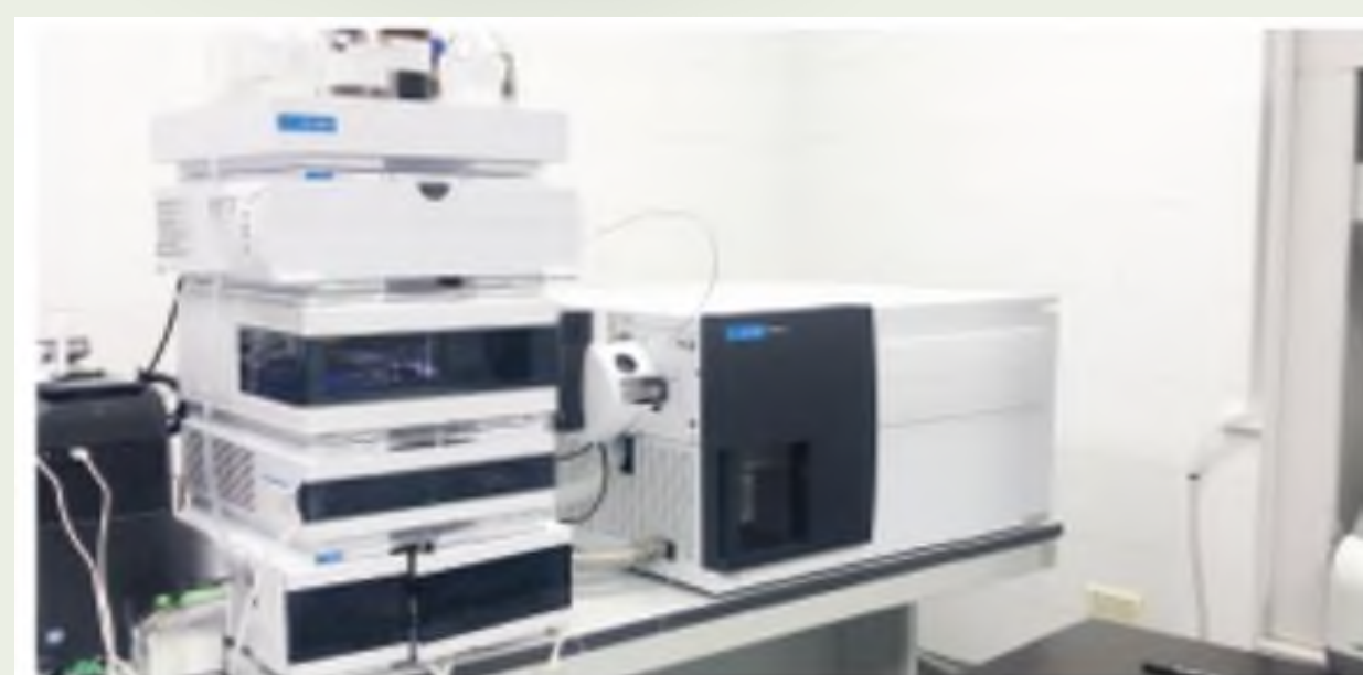
Хроматограф жидкостный Agilent 1260 Infinity II (SG2111G206) с Triple Quadrupole 6470 LC/MC System
