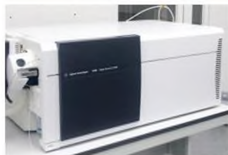
Хроматограф жидкостный Agilent 1260 Infinity (US83870021) с Triple Quadrupole 6460A LC/MS System
